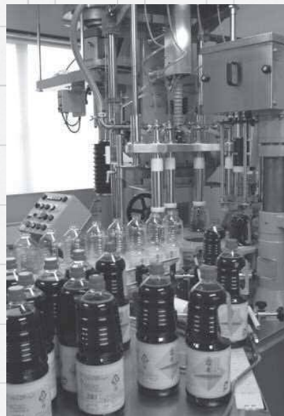
ひょうご産業活性化センターの支援を受けて導入した充填機
