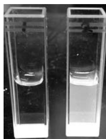
図1 セレニドの蛍光検出
