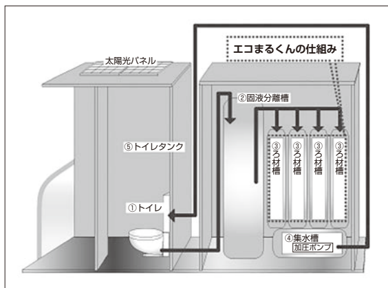
②空気を遮断したタンク内で糞・尿を分離し、③オリゴ糖ろ過材で浄化します
