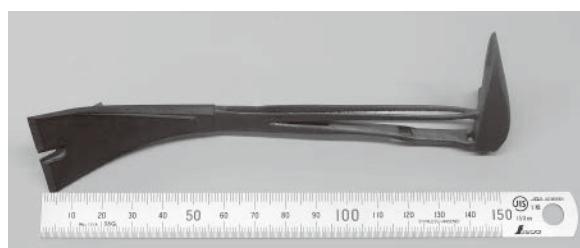
図2 トポロジー最適化適用後の三徳パール
