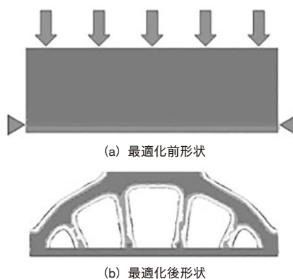
図1 トポロジー最適化を適用したブロック
