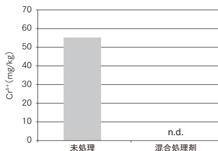
図2 混合処理剤による \text{Cr}^{6+} 生成抑制
