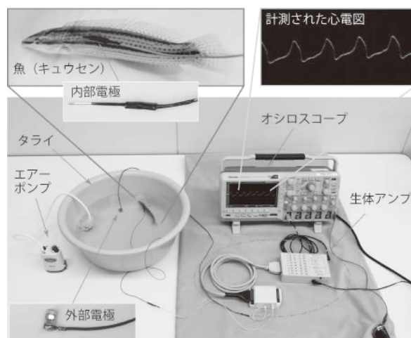
【図2】 実証実験に用いた生体電気計測システム等
