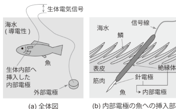
【図1】 海水を利用した新規生体電気計測手法
