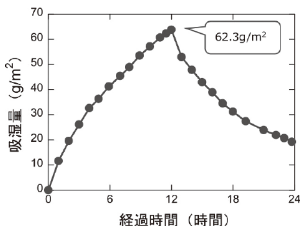
開発中の新「タツタイル」の吸放湿性
