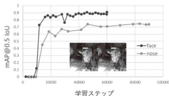
【図2】 学習曲線
