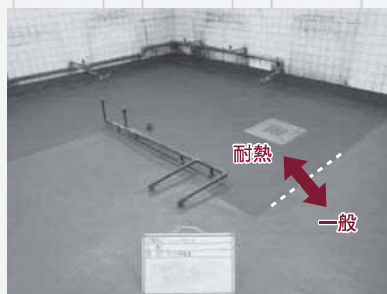
施工後(色の濃淡部分は、一般と耐熱仕様に分かれています)
