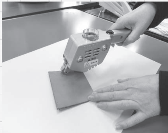
開発から手掛けたホットメルト糊付機
